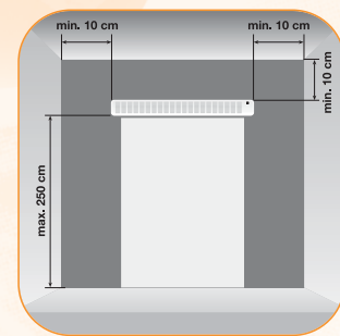
Установочные размеры
