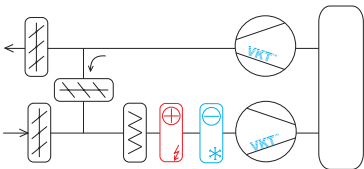
Схема 6.3 VAC-EF-ShD1D3D3D35D125TeKt
