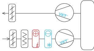
Схема 6.1 VAC-EF-ShD1D3D3D35D125TeKt
