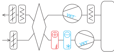
Схема 6.4 VAC-EF-ShD1D3D3D35D125TeKt
