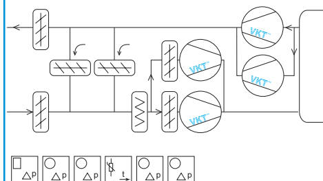
Схема 8.2 VAC-ShD1D3D3D3D35
