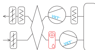
Схема 1.4 VAC-W-ShD1D3D3D35D125D14T123
