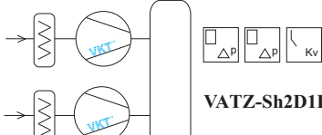
Схема 7.2 Воздушно-тепловая завеса с двумя вентиляторами
