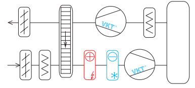
Схема 6.5 VAC-EF-ShD1D3D3D35D125TeKt
